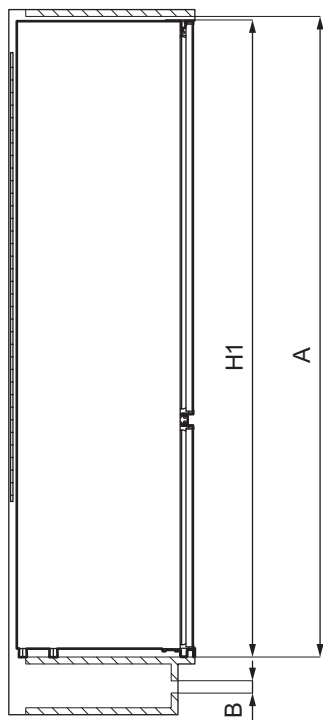
Габаритные размеры 1
