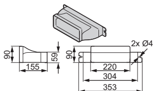
S11 M2CKCF26U Diffuser
