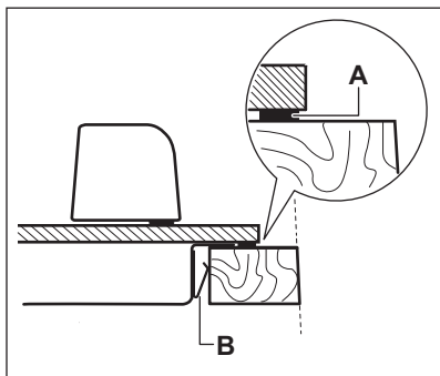
A) guarnizione in dotazione B) staffa montata
