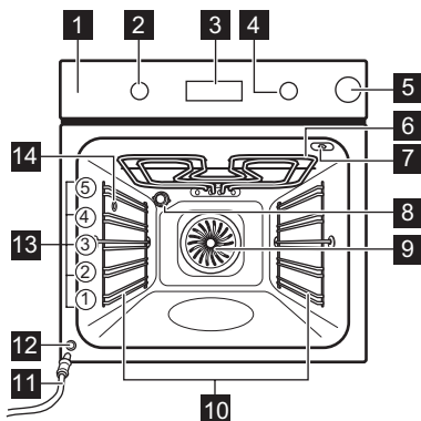
1 Vadības panelis
