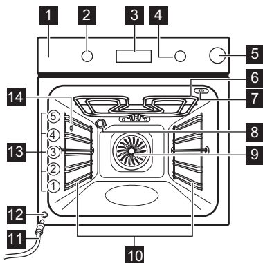
1 Панель управления
