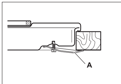
А) входящая в комплект поставки крепежная скоба
