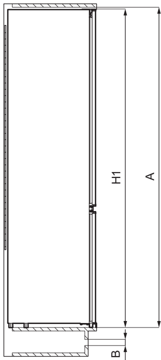
Utvendige dimensjoner 1
